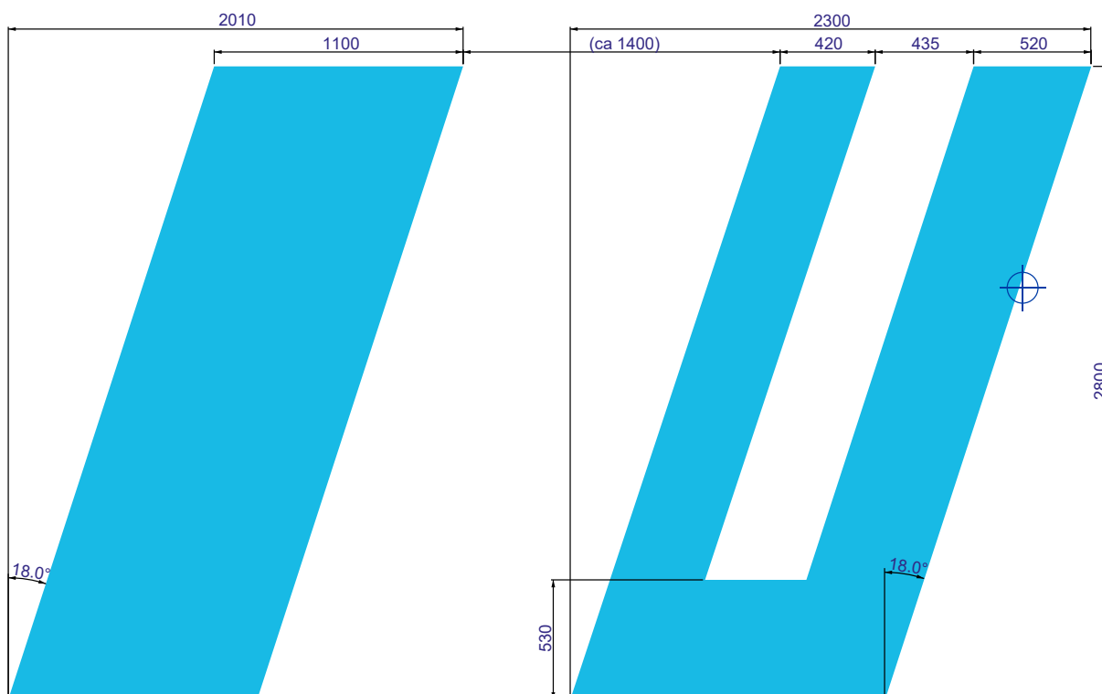
214 B. Dekormålning, höger sida, bak.
