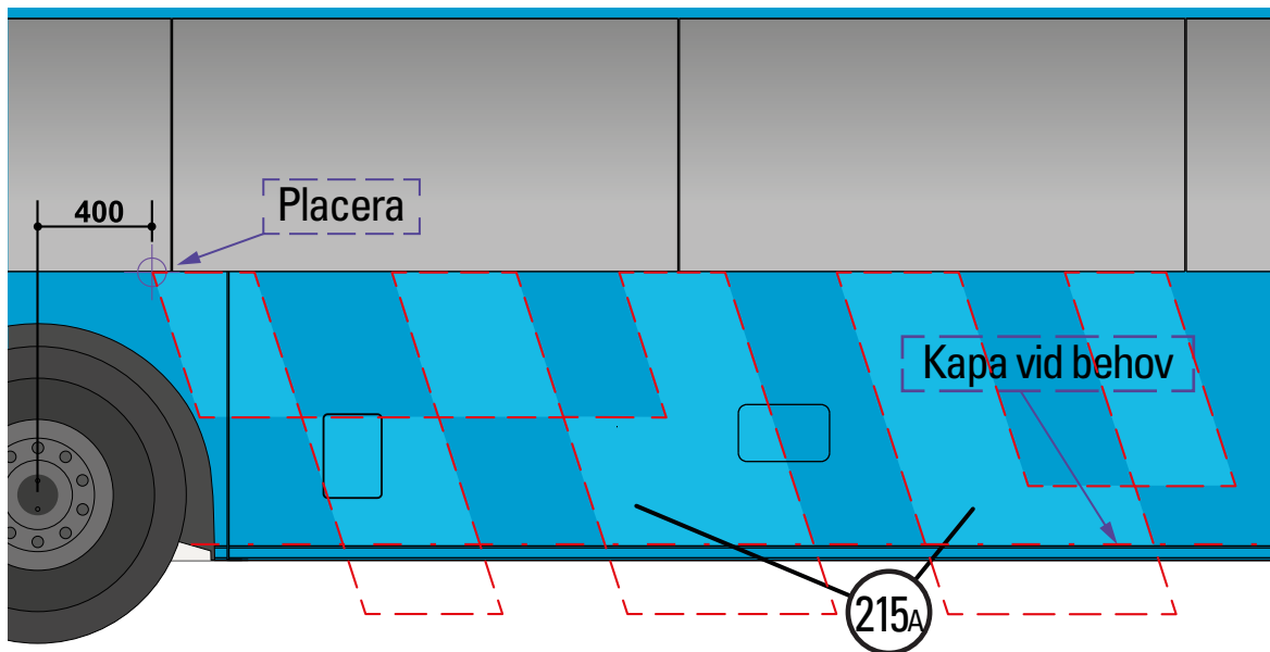
215A. Dekorfolie vänster sida fram
