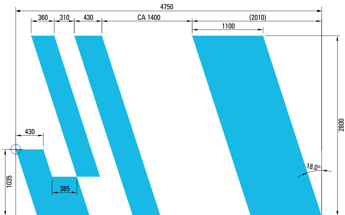
215 B. Dekormålning, vänster sida, bakre.
