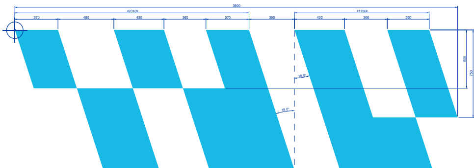
215 A. Dekormålning, vänster sida, främre.
